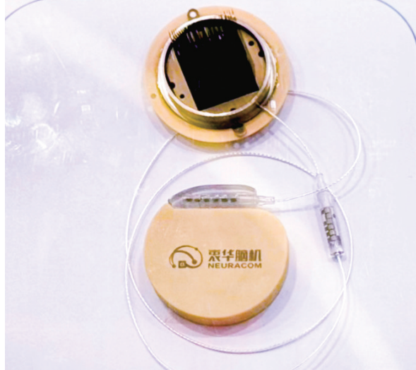
衷华脑机研发的高通量植入式脑机接口系统HIMA60000系列,其最大通道数达65536个,能精准“读脑”和“控脑”。
