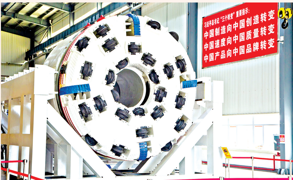
全球首台掘爆机在江夏研制成功。
